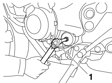
1. Clé dynamométrique
